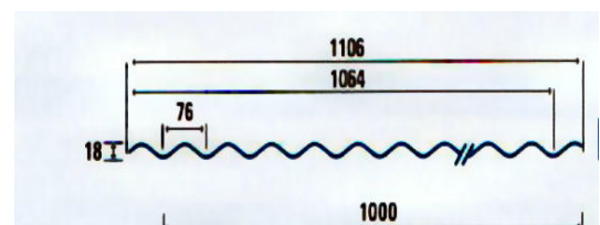
Sinus-/Wellenprofil
