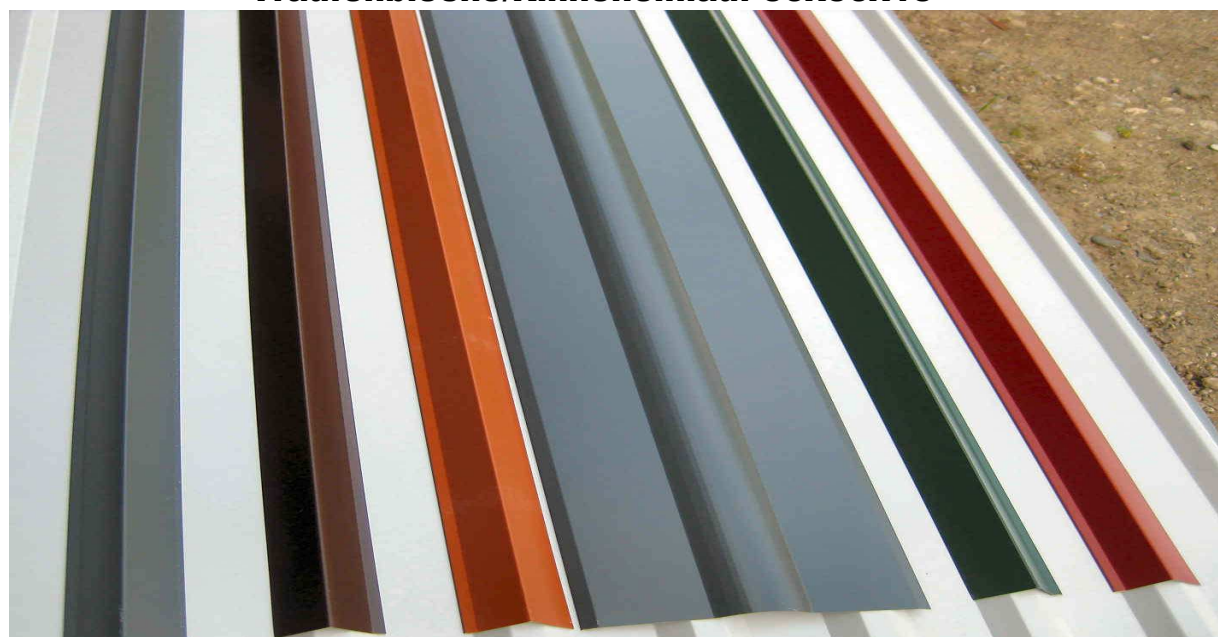
Kantenteile jeweils 2-m-lang – Verlegung überlappend (Nutzlänge ca. 1,90 bis 1,95m) Siehe auch Sonderkantenteile- Fertigung in eigener Produktion nach Kundenvorgabe
